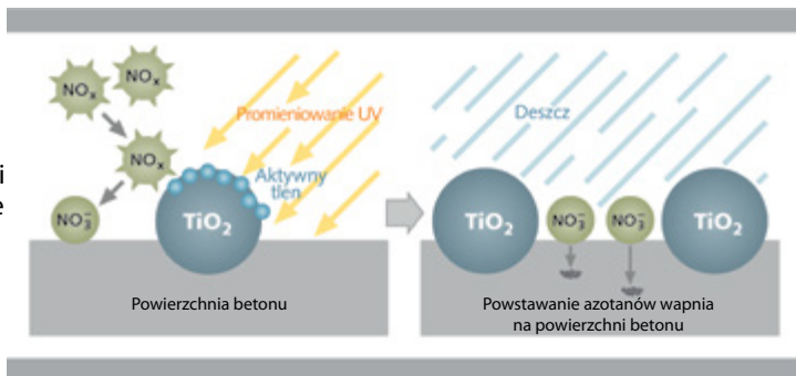
Mechanizm oczyszczania powietrza z tlenków azotu \text{NO}_x przez aktywną fotokatalityczną powierzchnię kostki brukowej wykonaną z użyciem cementu TioCem®
