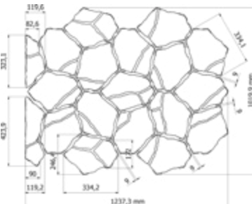
Ułożenie kostek Sasso
