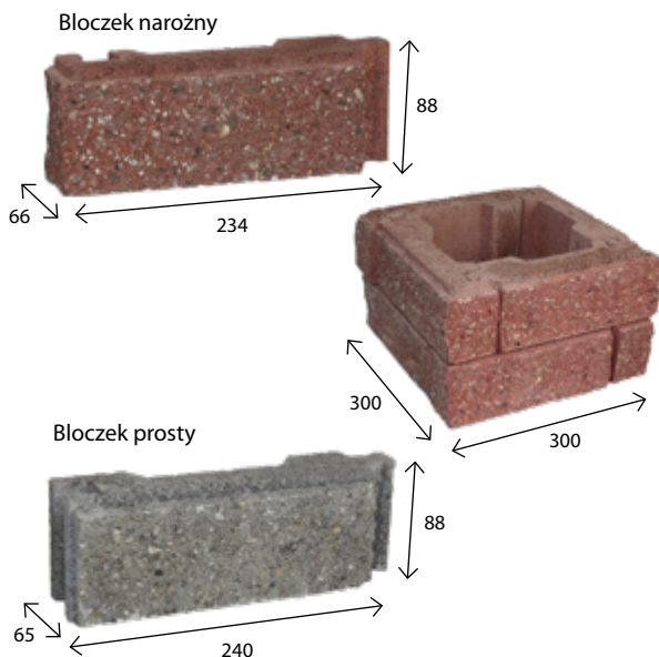
Bloczek prosty Legobet 8,8
