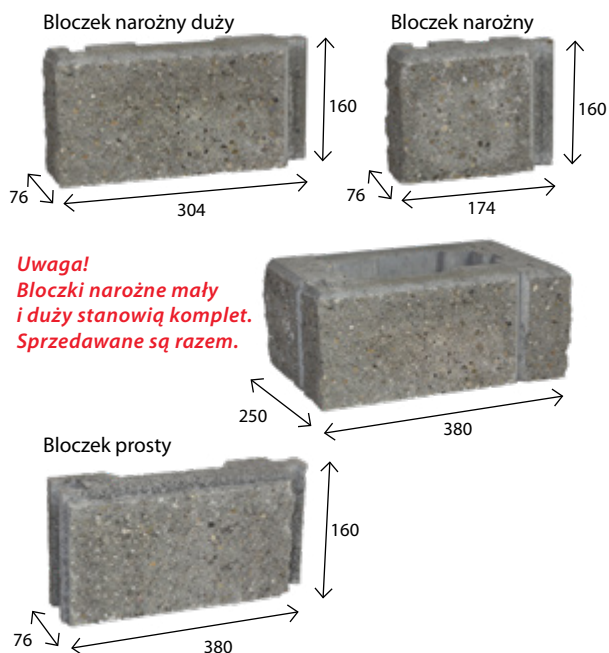
Bloczek prosty Legobet Grand
