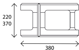
Bloczek cokołowy 370
