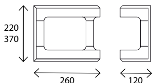
Bloczek słupkowy 370
