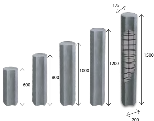
Palisada Rondo 100
