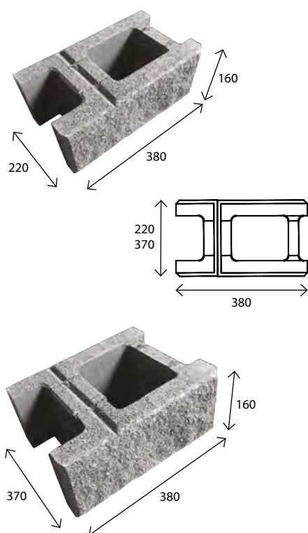
Bloczek cokołowy 370
