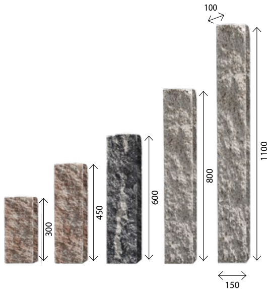
Palisada Cios Skalny 45
