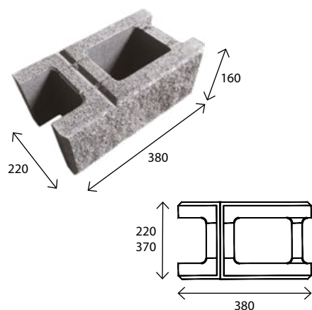
Bloczek cokołowy 370
