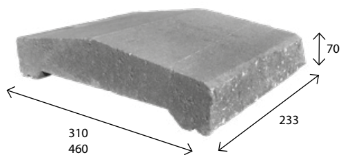
Daszek Orawa 370
