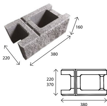
Blocek cokołowy 370
