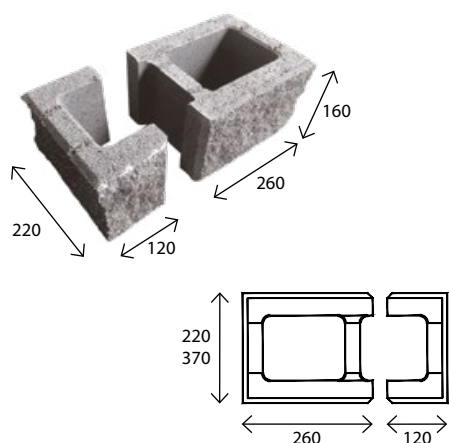
Blocek słupkowy 370
