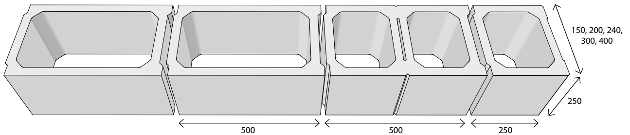
Pustak półkowy pakowany 1szt/warstwę
