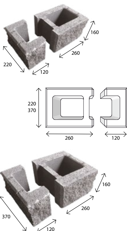
Bloczek słupkowy 370
