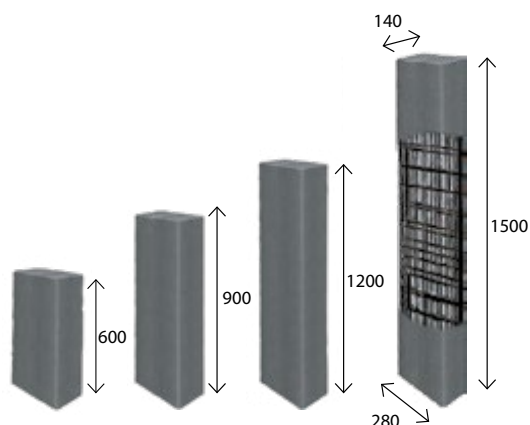
Palisada prostokątna 120
