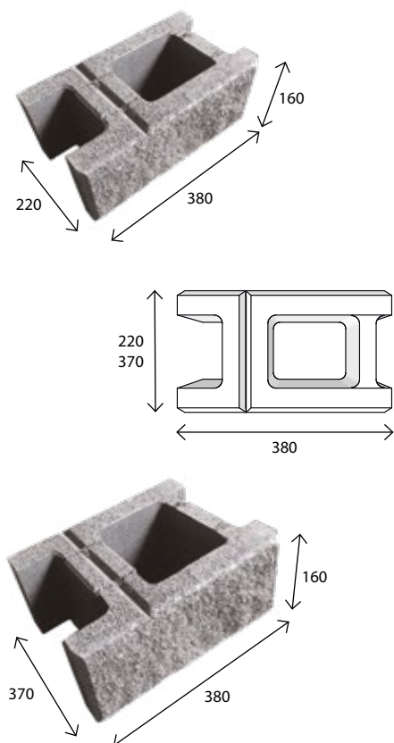
Bloczek cokołowy 370
