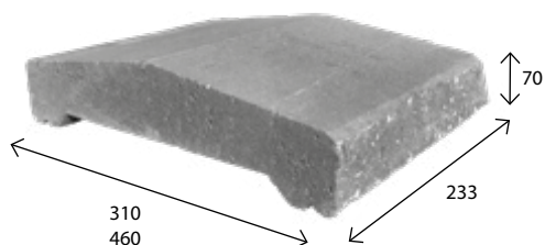
Daszek Orawa 370
